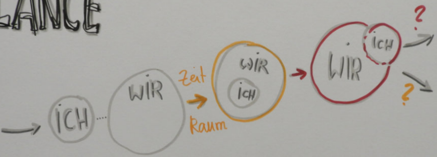
Abb 5: Integration & Differenzierung - ergebnis offen
